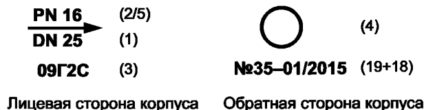
Рисунок Г.4 — Пример расположения маркировки обязательными знаками на корпусе обратного клапана
