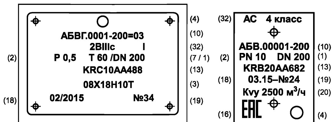
Табличка на герметическом клапане для АС, 2-й класс безопасности
