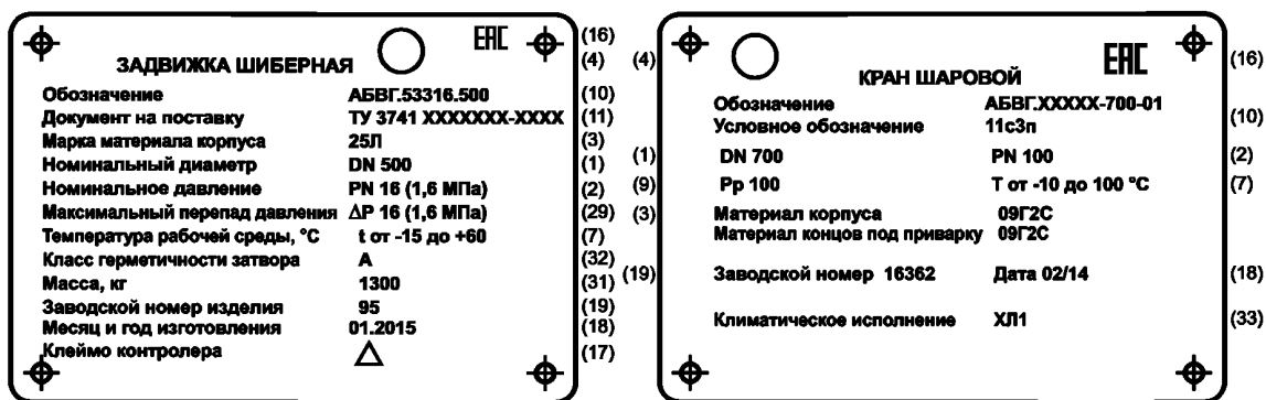
Табличка на шиберной задвижке
