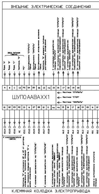
Блок схема ШУ з.п. ПС 52 местное+дистанционное управление+обр связь. U иш =230VAC
