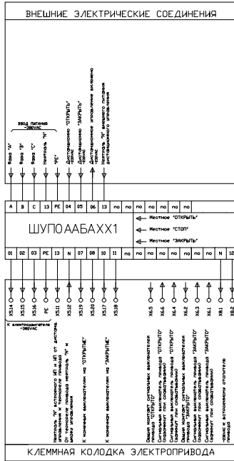
Блок схема ШУ з.п. ПС 52 местное+дистанционное управление+обр связь. U иш =24VDC
