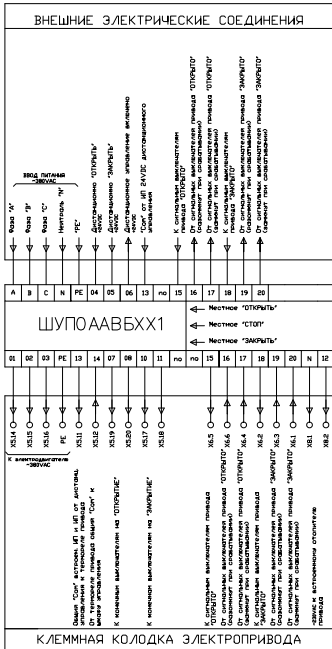
Блок схема ШУ з.п. ПС 52 местное+дистанционное управление+обр связь. U иш =24VDC
