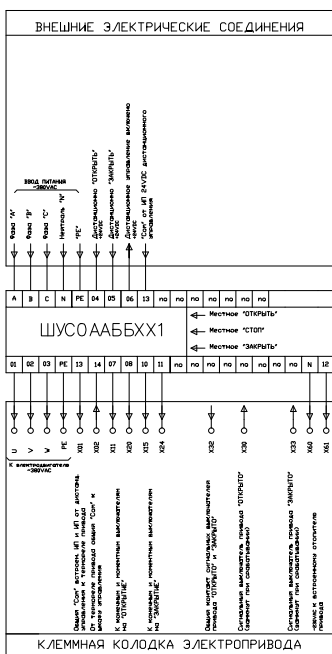
Блок схема ШУ э.п. АР-МОК 63 местное+дистанционное управление. U_{ном}=24VDC
